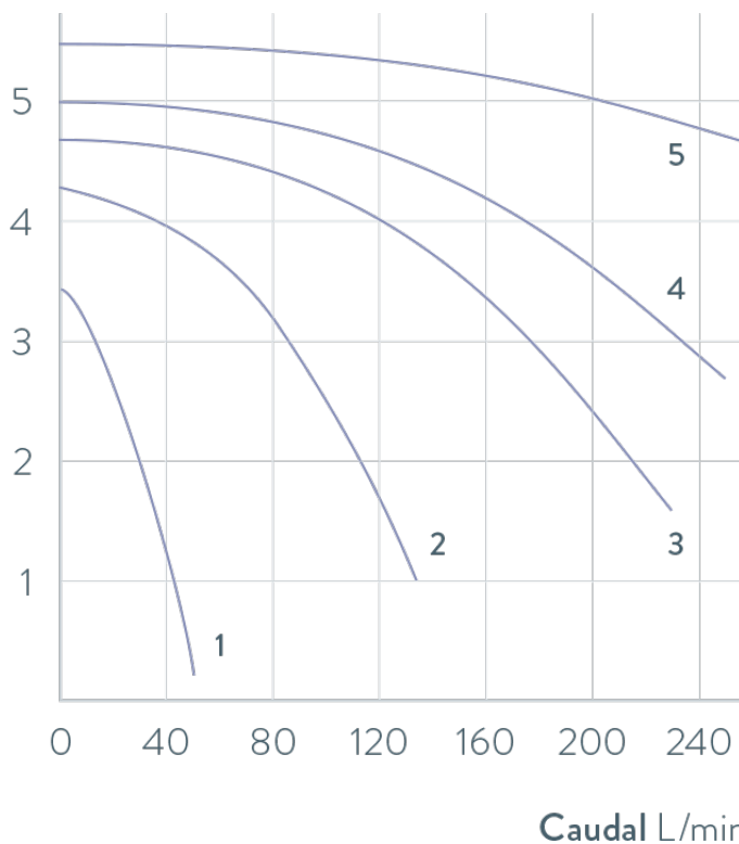
CURVAS CARACTERÍSTICAS DE LAS BOMBA Bombas estándar (3 bar), 50 Hz; Líquido caloportador: Agua Presión bar
